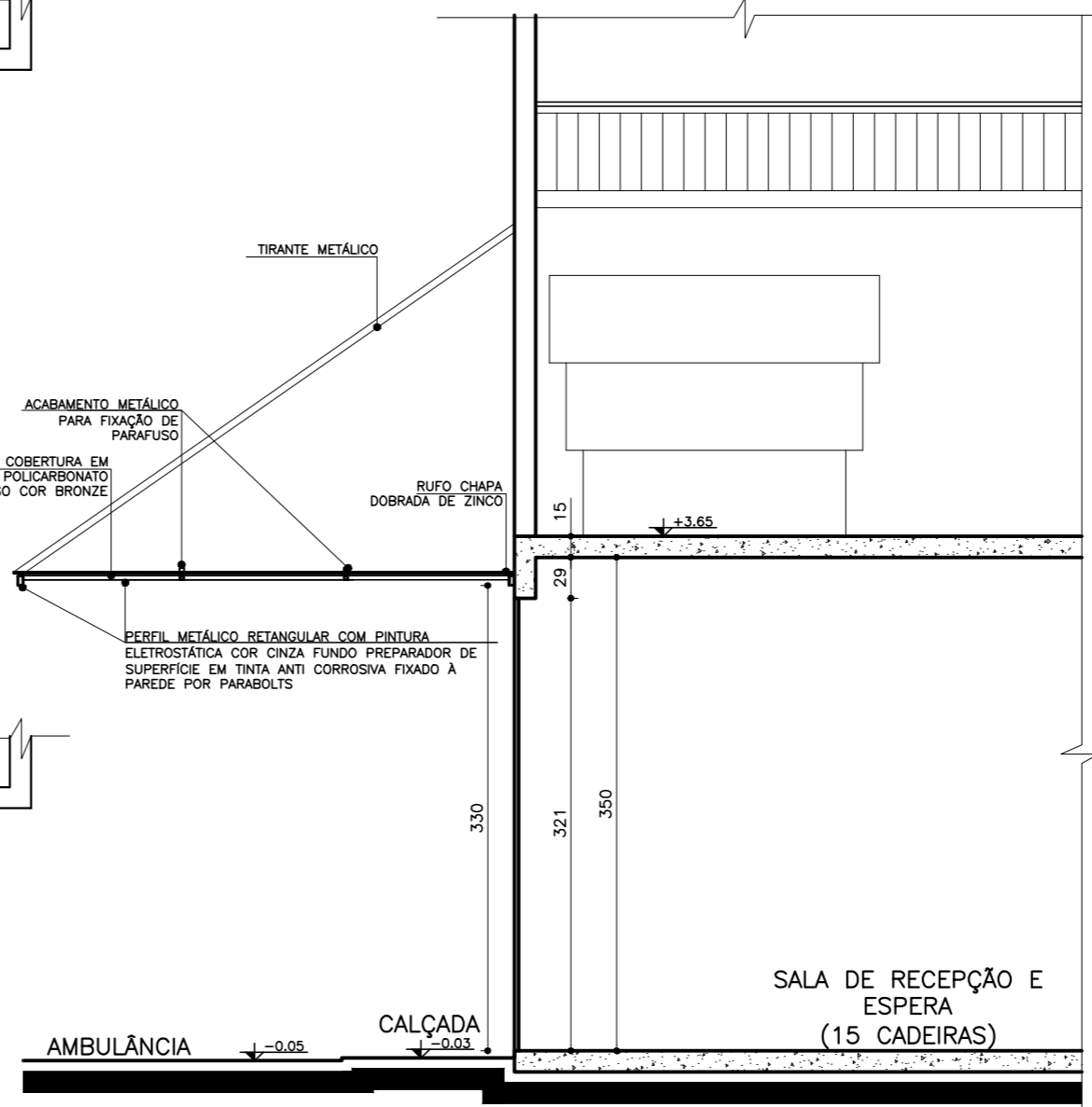
03 Seção A'- Marquise Entrada Principal Esc.: 1:50
