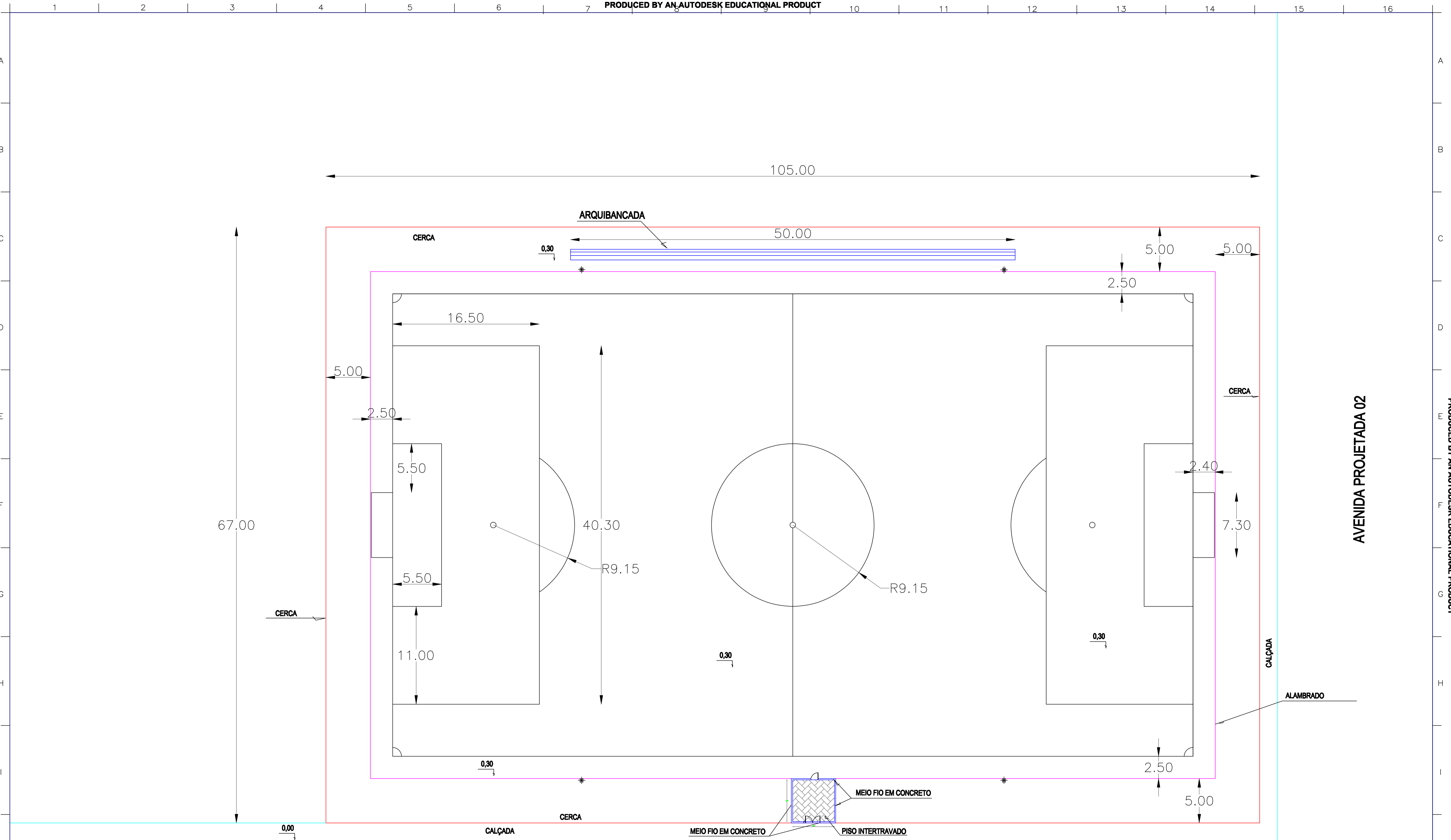
RUA PROJETADA 23 ESCALA - 1:200
