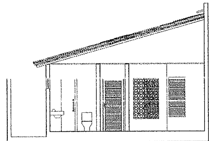
CORTE BB
