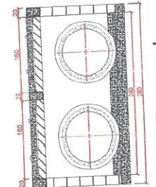
Corte Transversal
