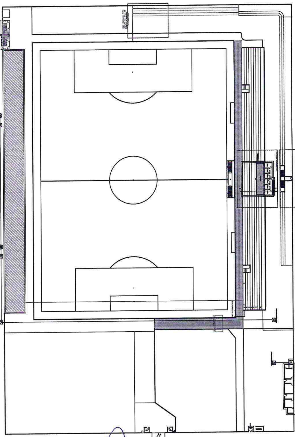
01 PLANTA BAIXA GERAL DO EDIFÍCIO ESCOLA
